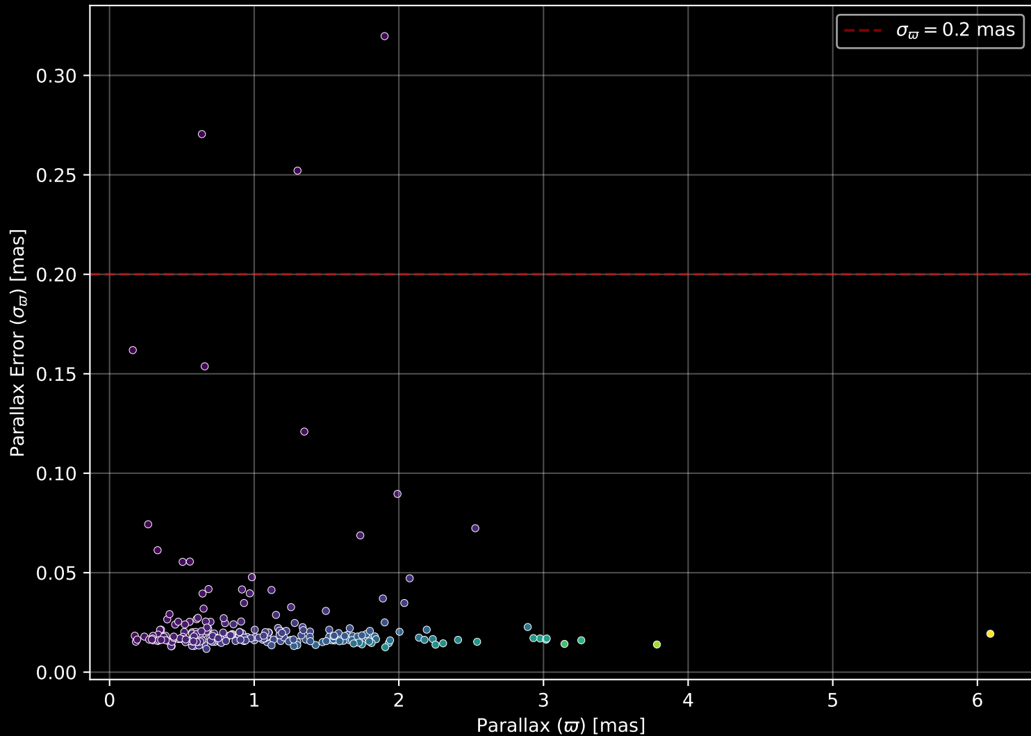
GALAH DR4 Field: [9332] Parallax Quality (n= 233)
