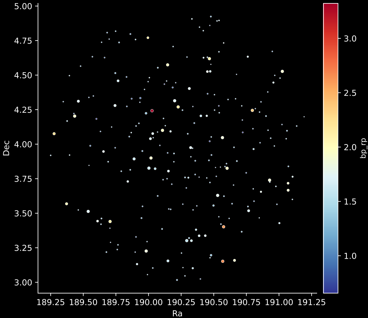
GALAH DR4 Field: [9332] Stars: 233
