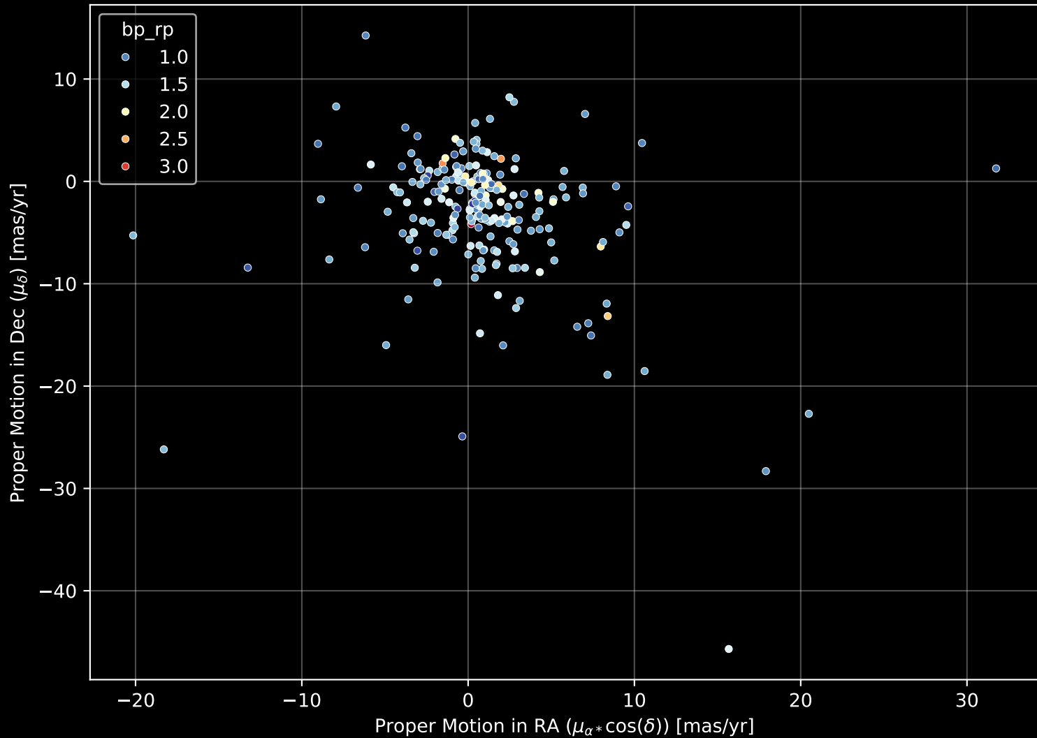
GALAH DR4 Field: [9332] Proper Motion Diagram (n= 233)
