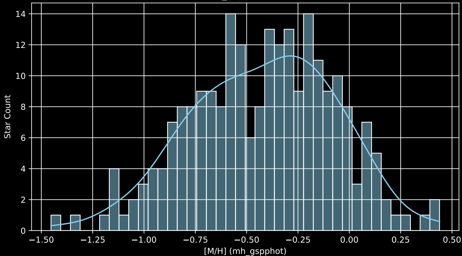
GALAH DR4 Field: [9332] [M/H] (mh_gspphot) (n= 231)
